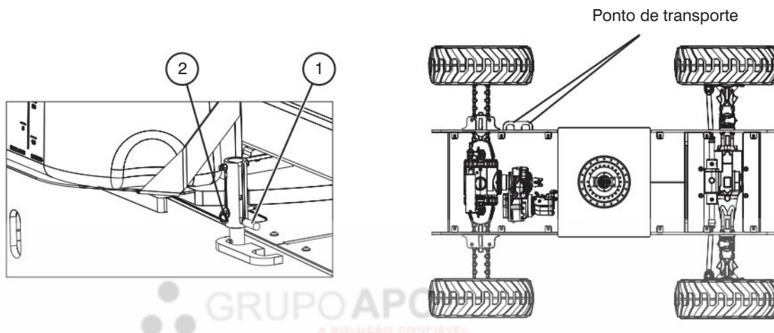
Figura 3-7. Trava de transporte da torre e pontos de travamento
